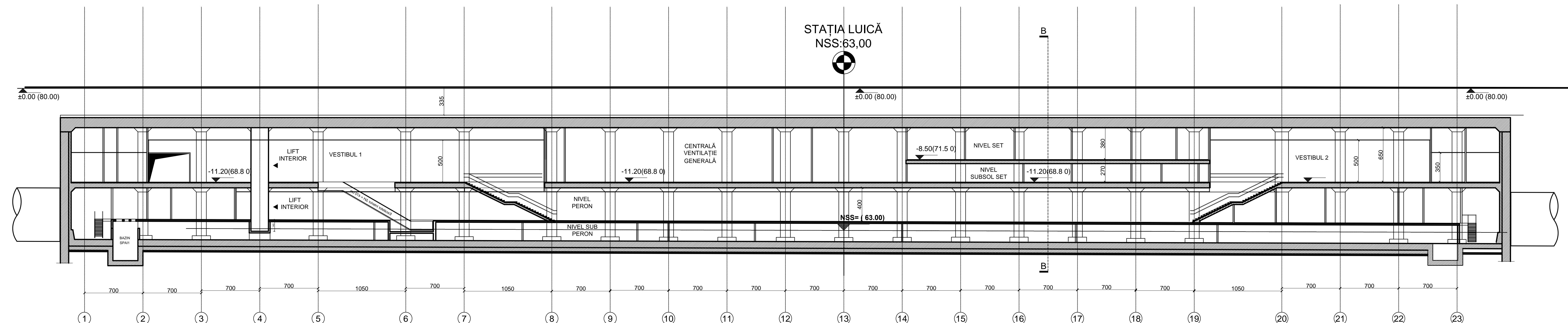
SECȚIUNE LONGITUDINALĂ A-A
