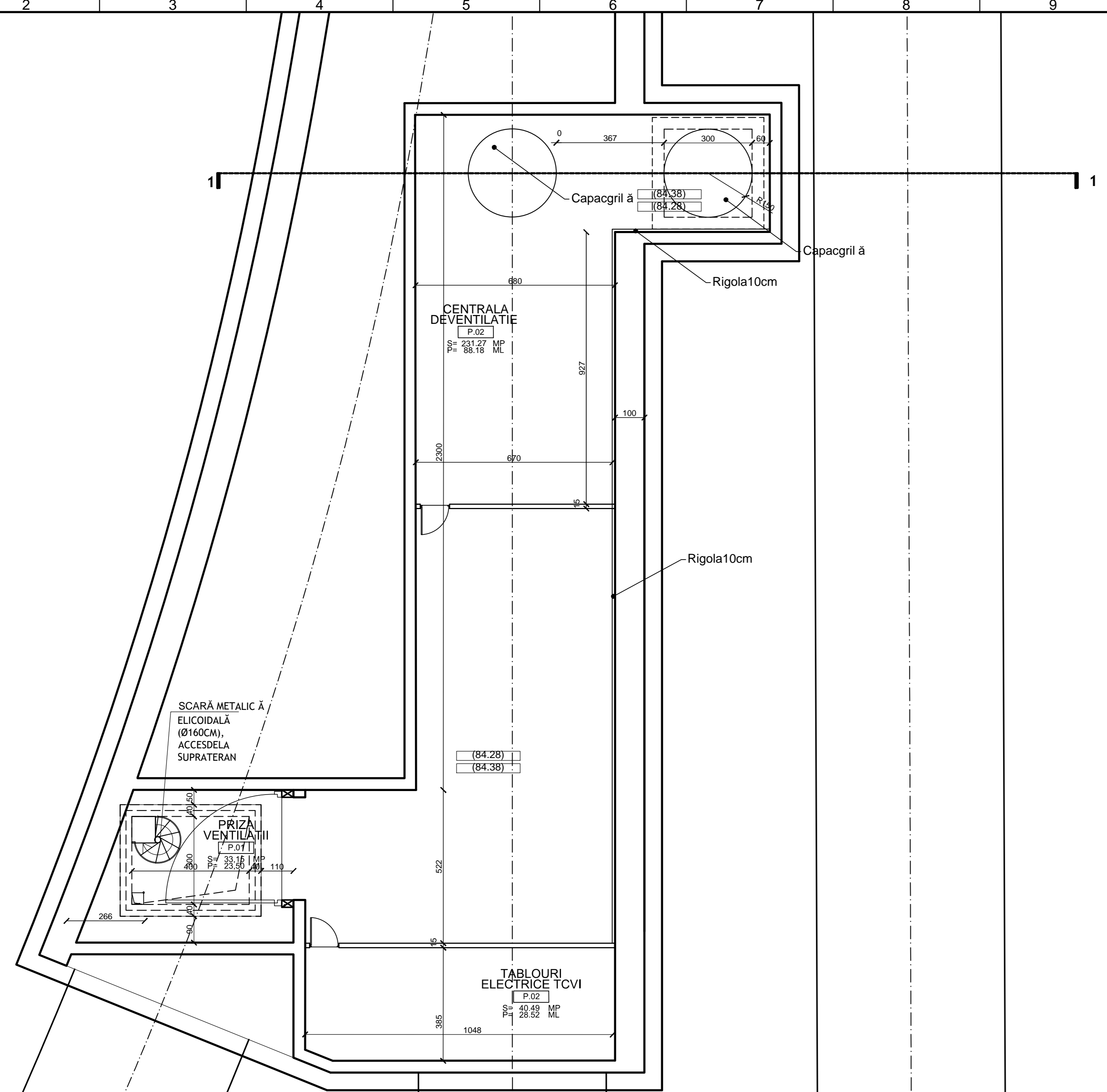
PLAN CENTRALA VENTILATIE INTERSTATIE sc. 1: 100
