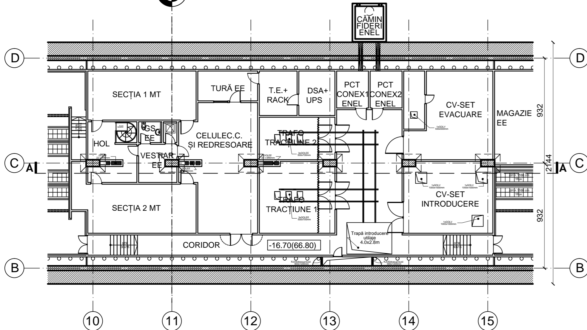
PLAN NIVEL SET
