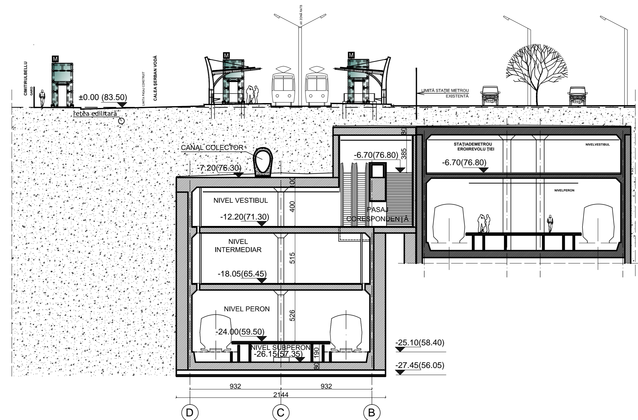
SECȚIUNE TRANSVERSALĂ B-B
