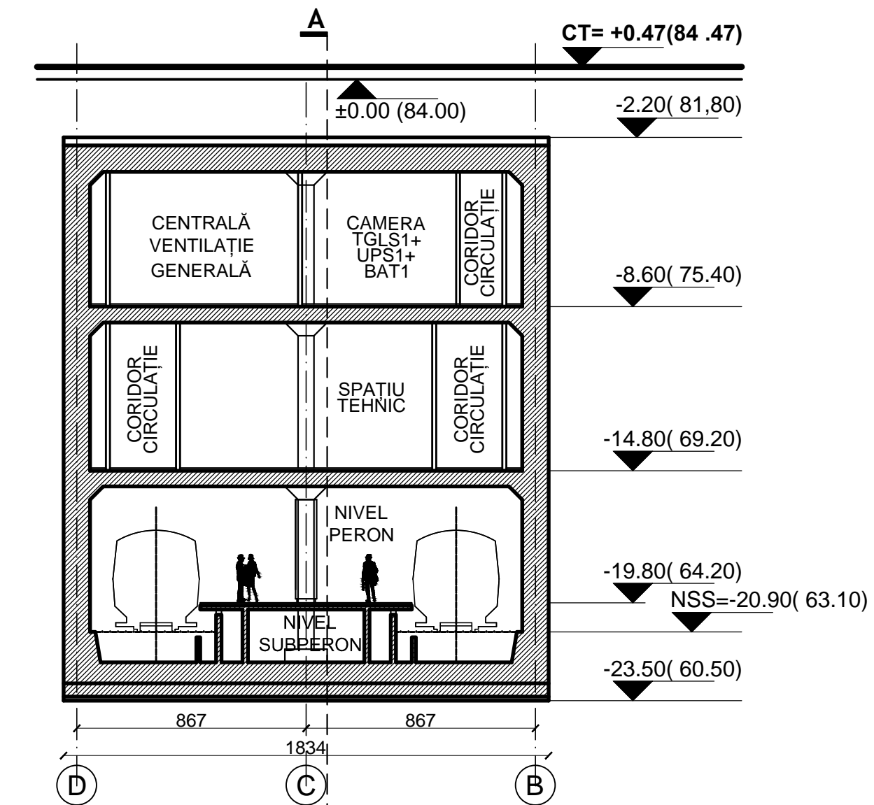
SECȚIUNE TRANSVERSALĂ B-B
