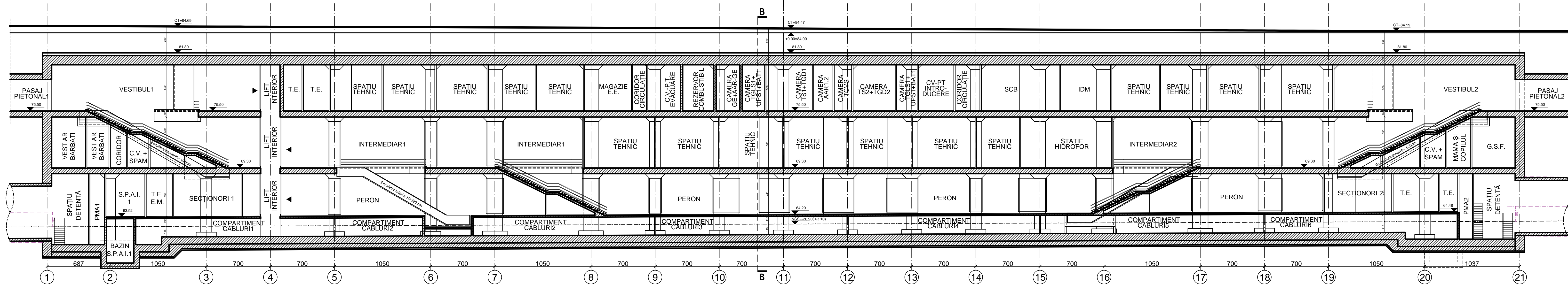
SECȚIUNE LONGITUDINALĂ A-A
