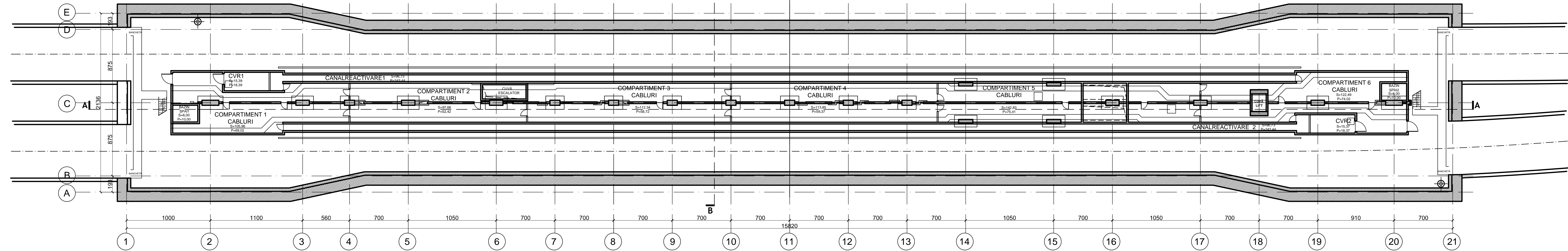
PLAN NIVEL SUBPERON
