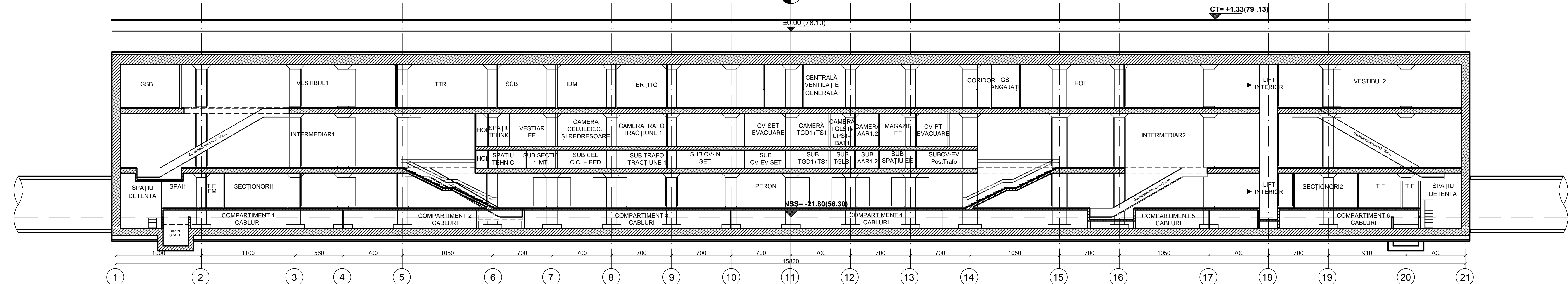
SECȚIUNE LONGITUDINALĂ A-A
