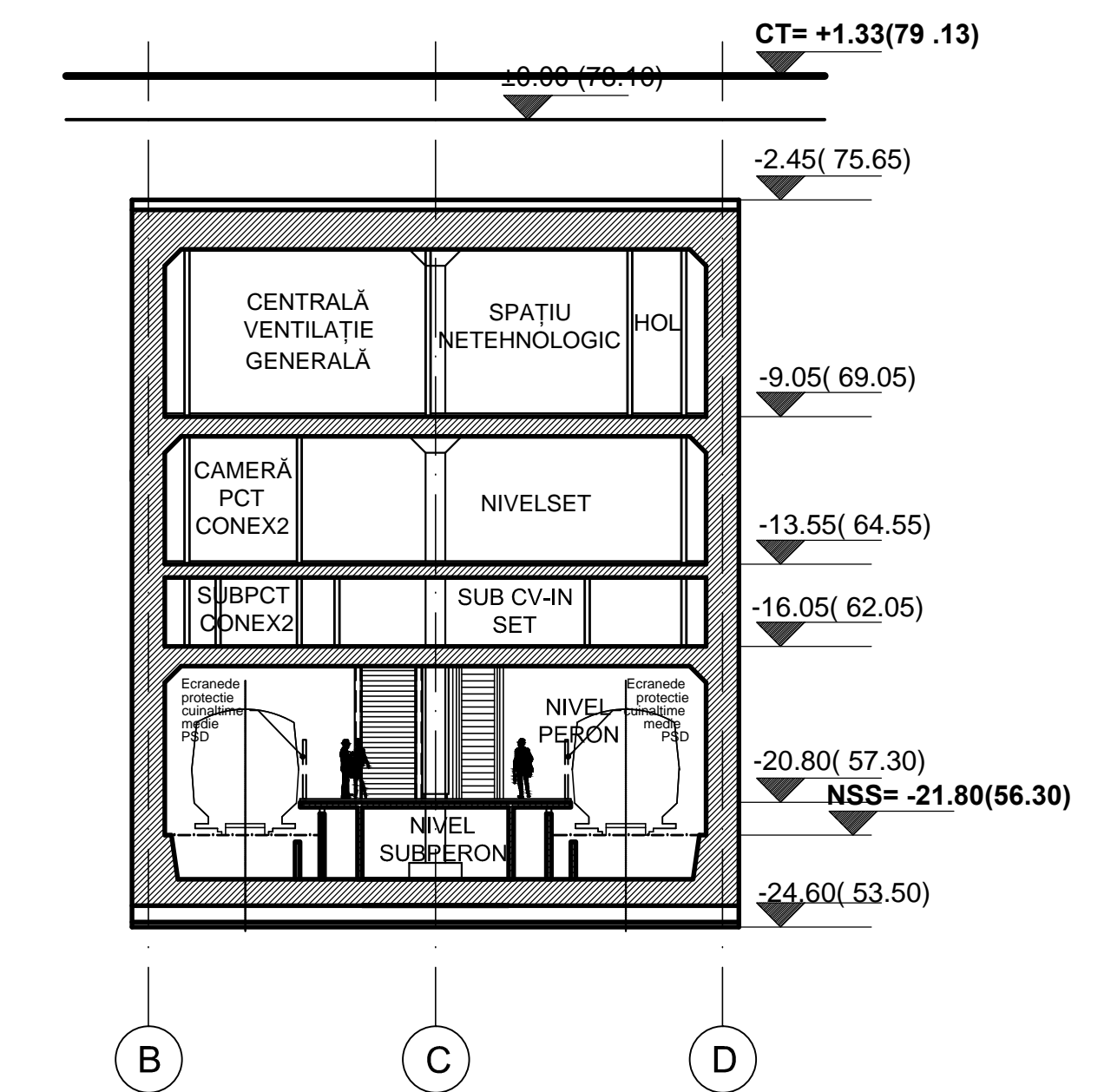
SECȚIUNE TRANSVERSALĂ B-B
