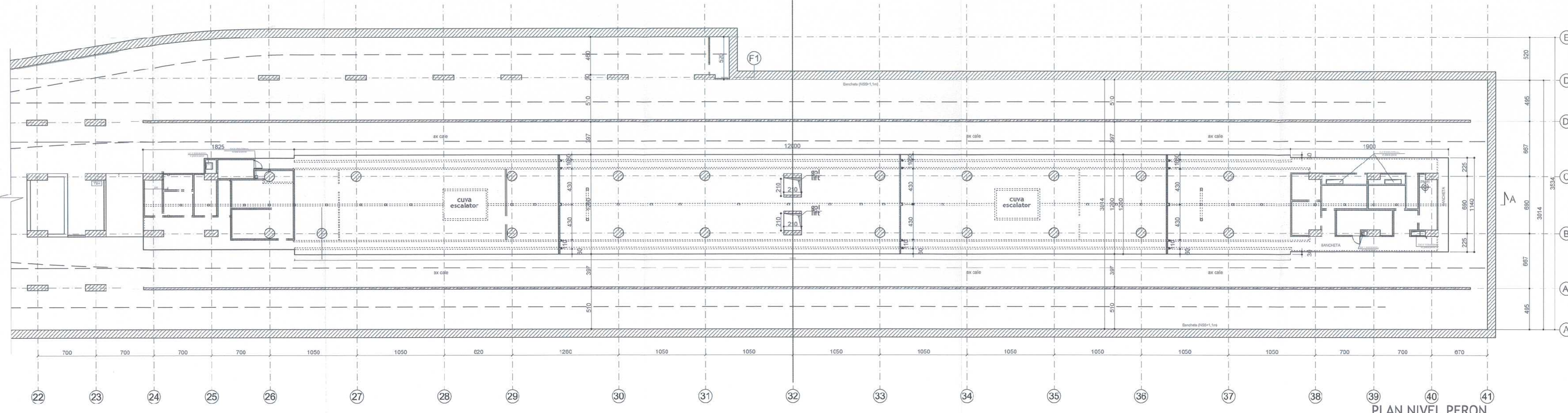
PLAN NIVEL PERON
