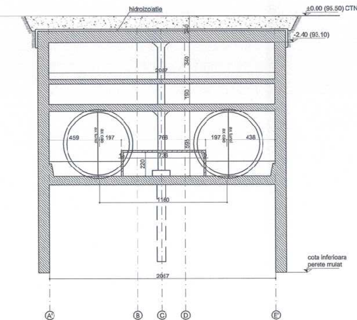
SECTIUNE TRANSVERSALA CURENTA A-A SCARA 1:200
