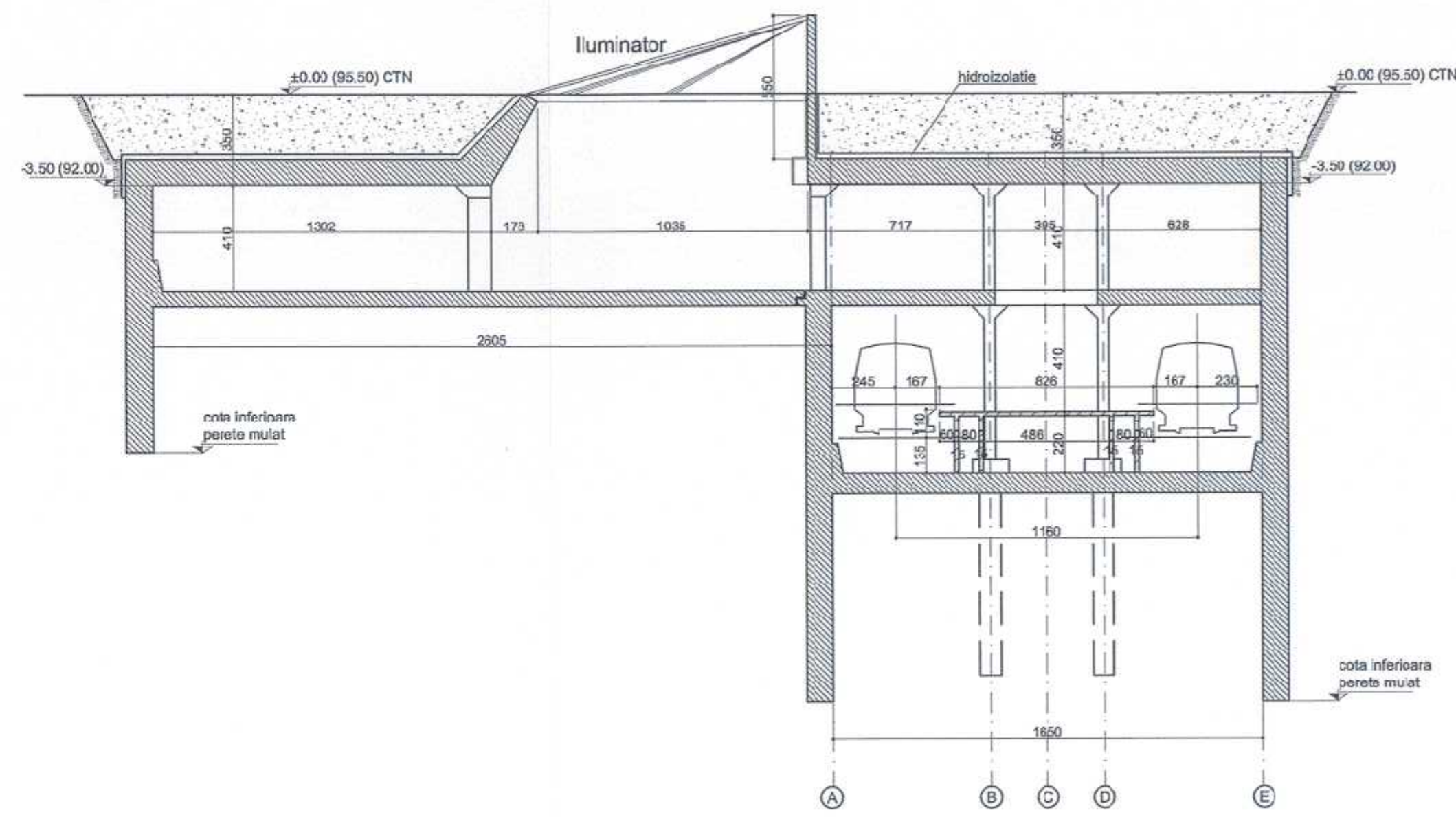
SECTIUNE TRANSVERSALA CURENTA B-B SCARA 1:200
