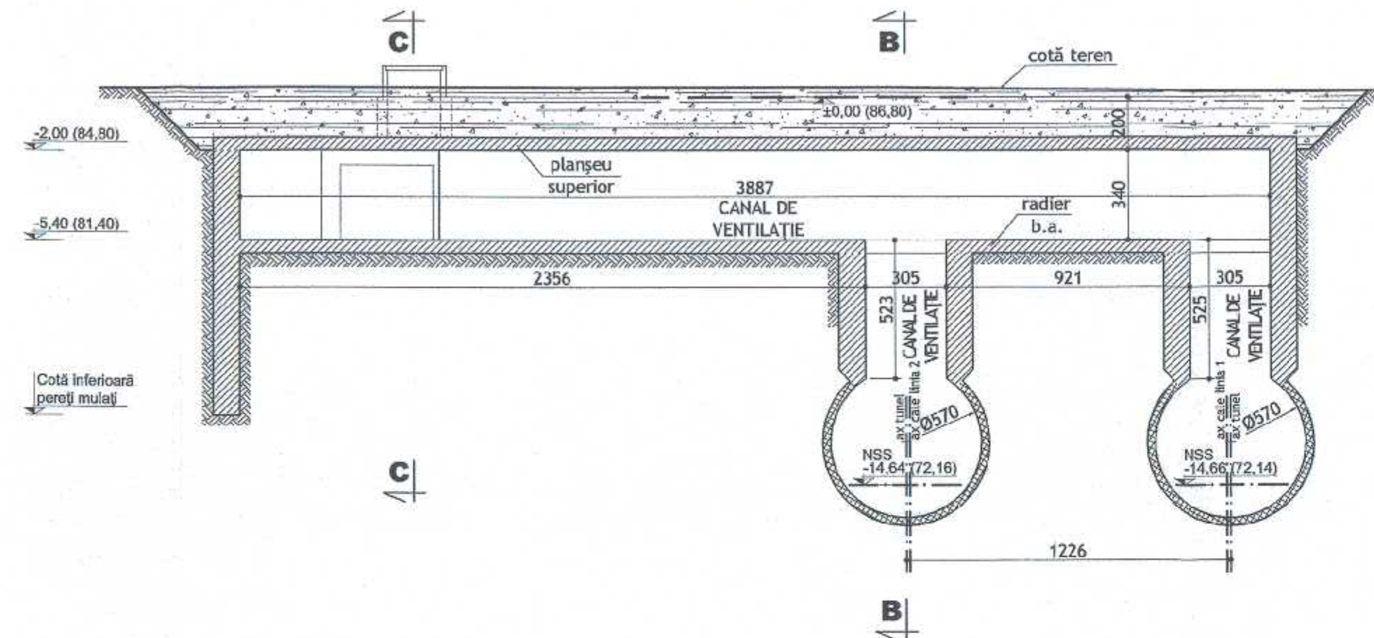
SECȚIUNEA A-A SCARA 1:200
