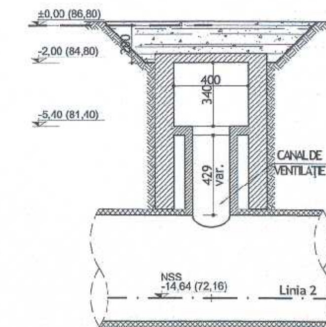
SECȚIUNEA B-B SCARA 1:200
