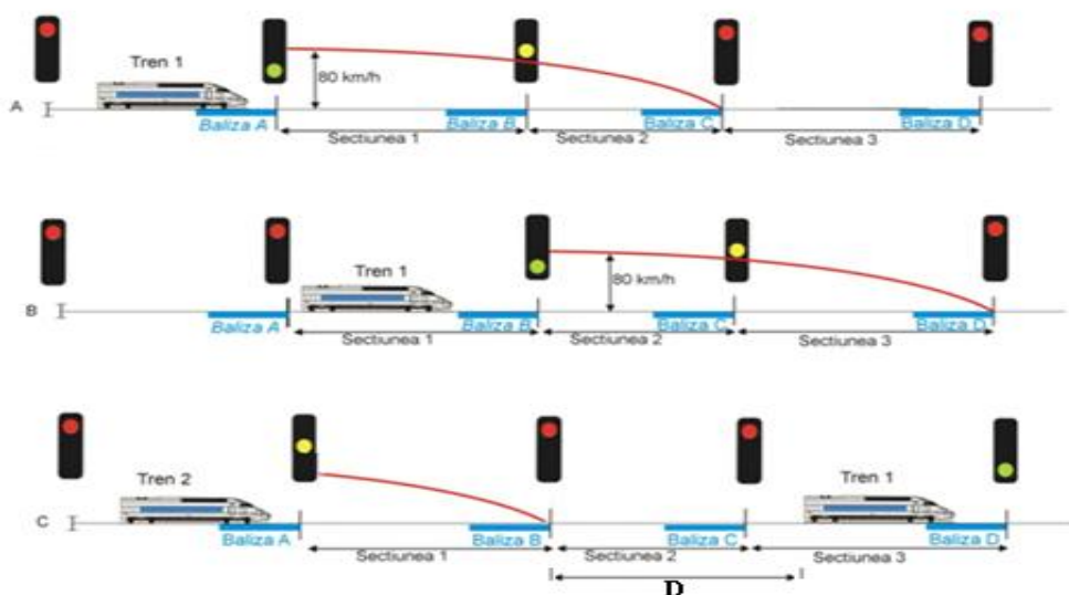
nivel 1 CED și BLA
